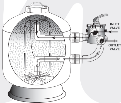
Waterco GFK-Filterkessel mit Seitenanschluss
