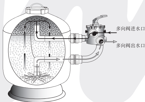
运水高侧装砂缸
