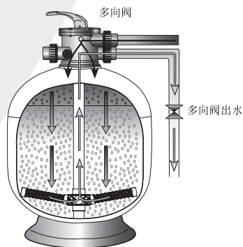
运水高顶装砂缸
