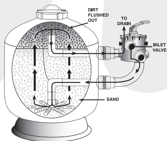
Factres Waterco à fibres de verre à montage latéral
