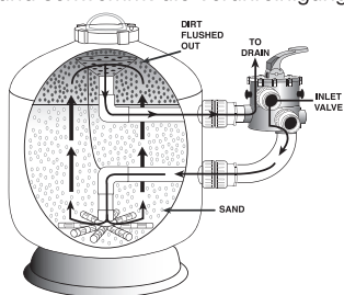
Waterco GFK-Filterkessel mit Seitenanschluss
