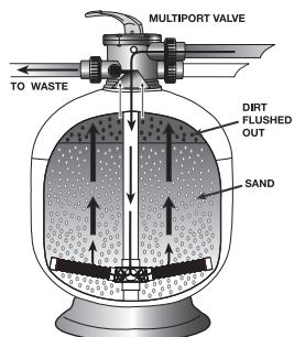
Factres Waterco à fibres de verre à montage par le haut
