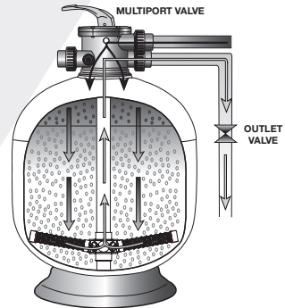
Waterco GFK-Filterkessel mit Obenanschluss
