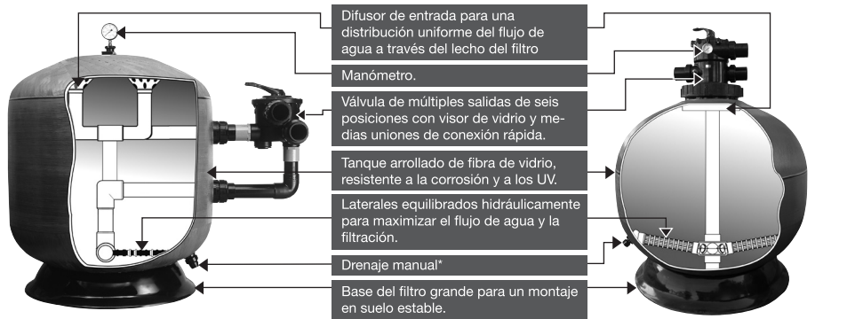
Filtros de fibra de vidrio de montaje lateral Waterco.
